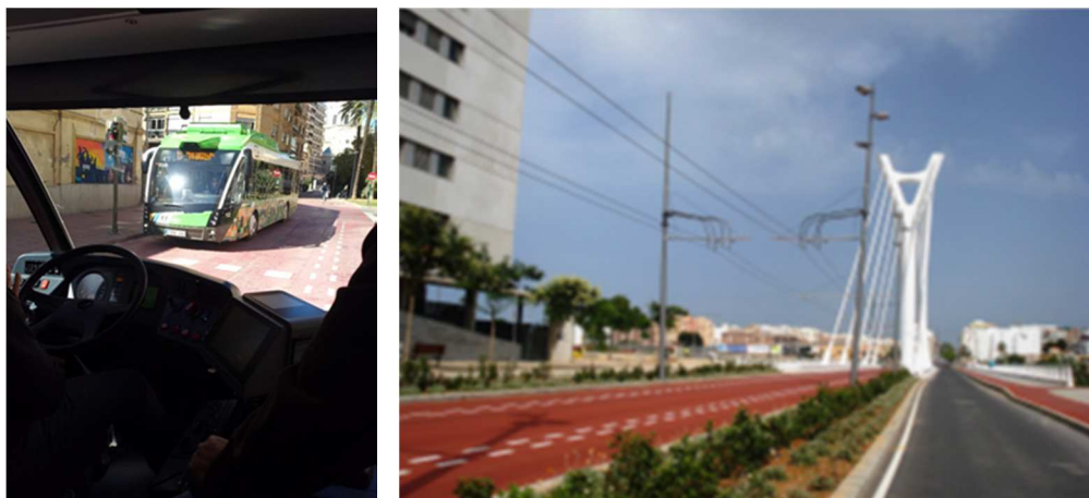
Figura 4. Exemplo materialização da linha de trajetória e dos limites do gabarit livre de obstáculos em Castellón (Espanha)
