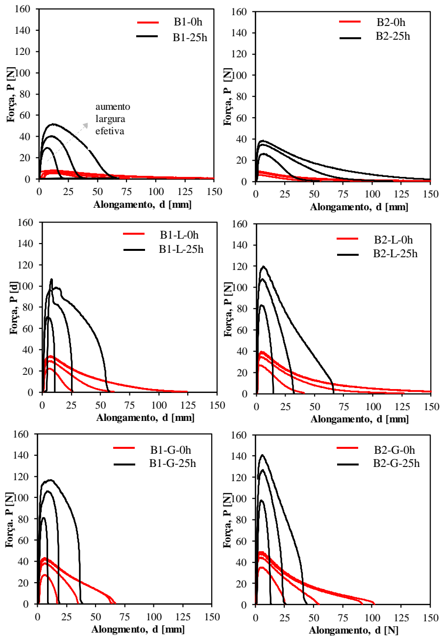
Fig.7. Resultados do ensaio de tração com diferentes dimensões de largura efetiva: betume B1 (à esquerda); betume B2 (à direita).
